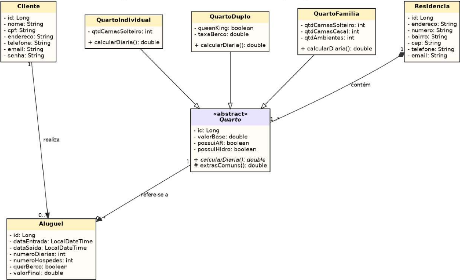
Diagrama de Classes – Sistema de Hospedagem Maraú
